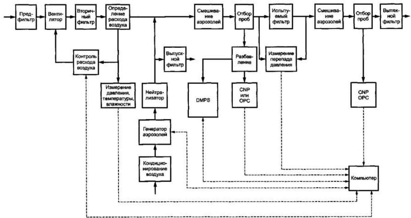
Рисунок 4 - Схема установки для испытания фильтров на эффективность статическим методом
