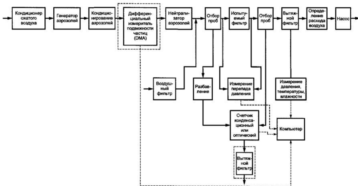
Рисунок 1 - Схема установки для испытаний фильтрующих материалов
