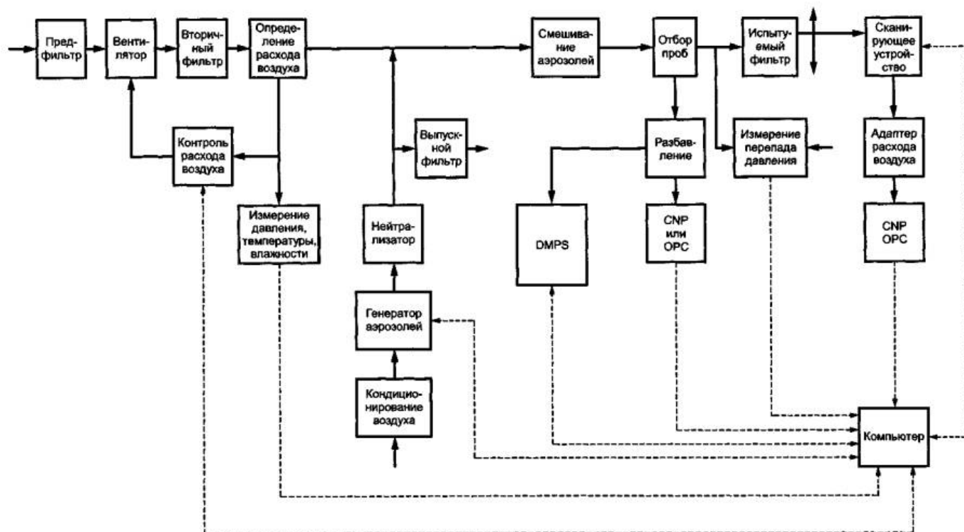
Рисунок 3 - Схема установки для испытаний фильтров на проскок (утечку)
